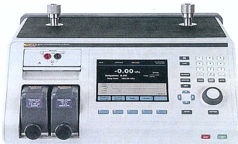
Рисунок 1 - Общий вид калибратора 2271А
