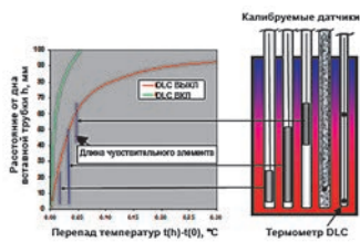
Рис. 5. Задание температуры. Система компенсации загрузки термостаата DLC
